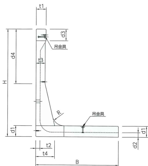
A-A断面図
