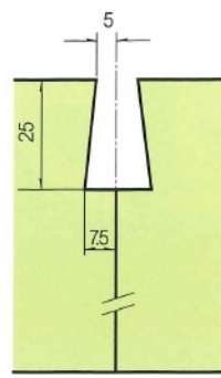
目地詳細図
