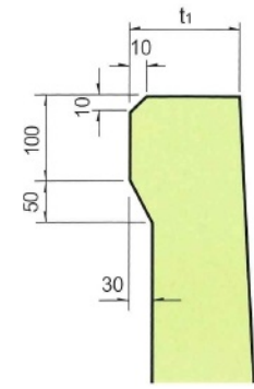
側壁頂部詳細図
