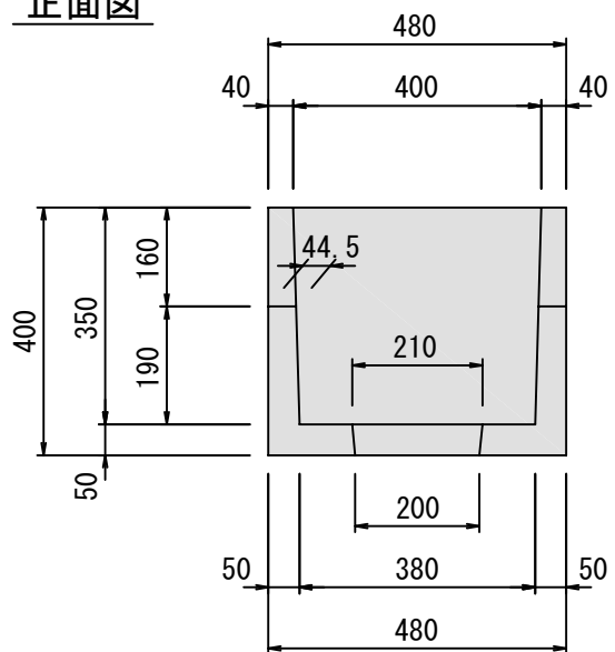
正面図
